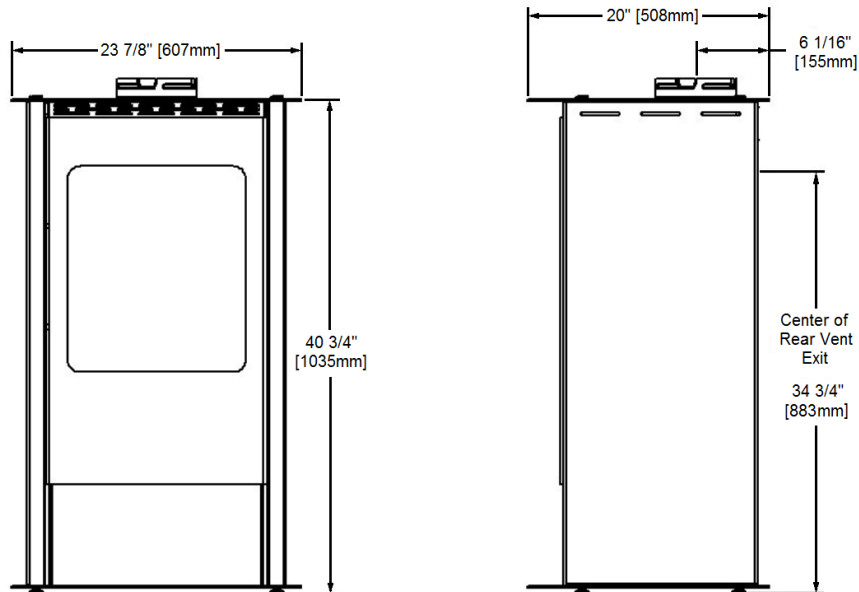
EUROPA Dimensions
